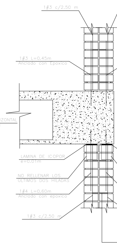
SECCIÓN B-B ESC 1:12.5
