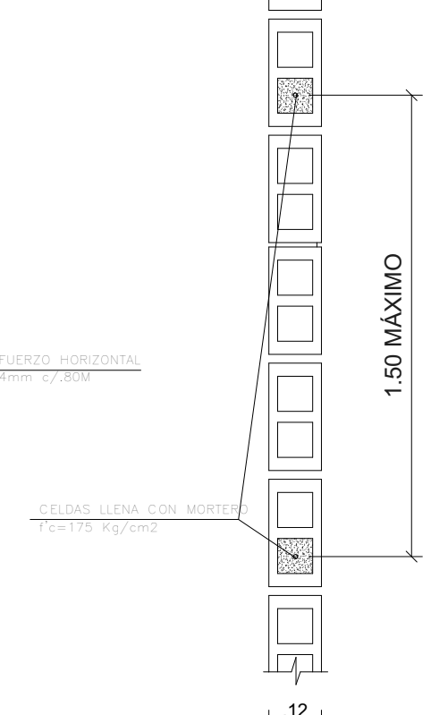
SECCIÓN C-C ESC 1:12.5
