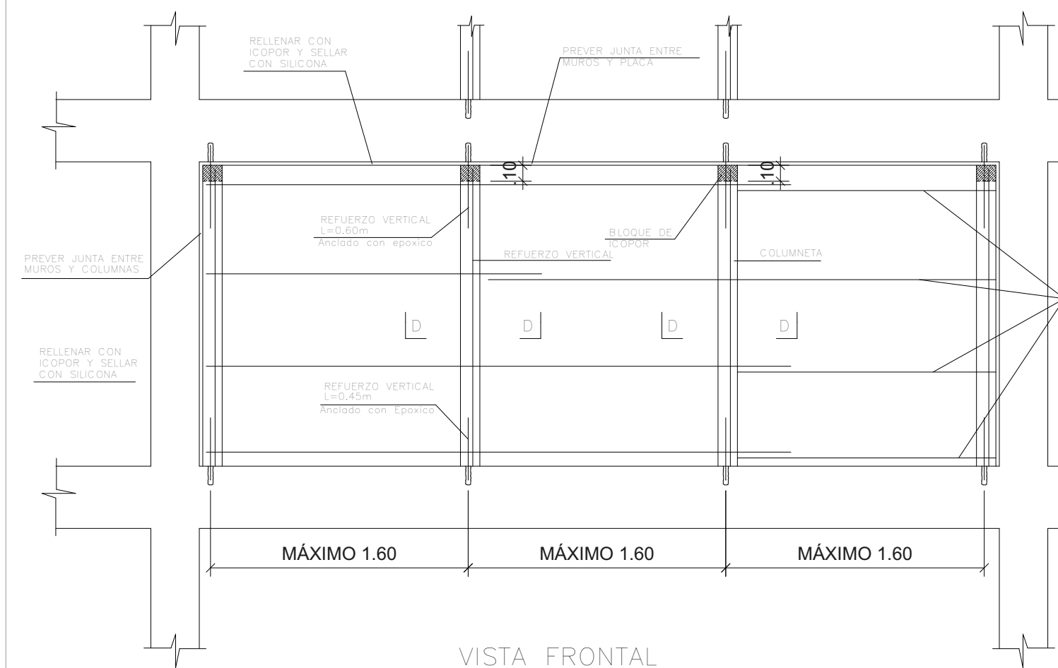
VISTA FRONTAL REFUERZO TÍPICO DE MUROS DIVISORIOS DE ALTURA TOTAL EN BLOQUE DE PERFORACIÓN HORIZONTAL ESC 1:25
