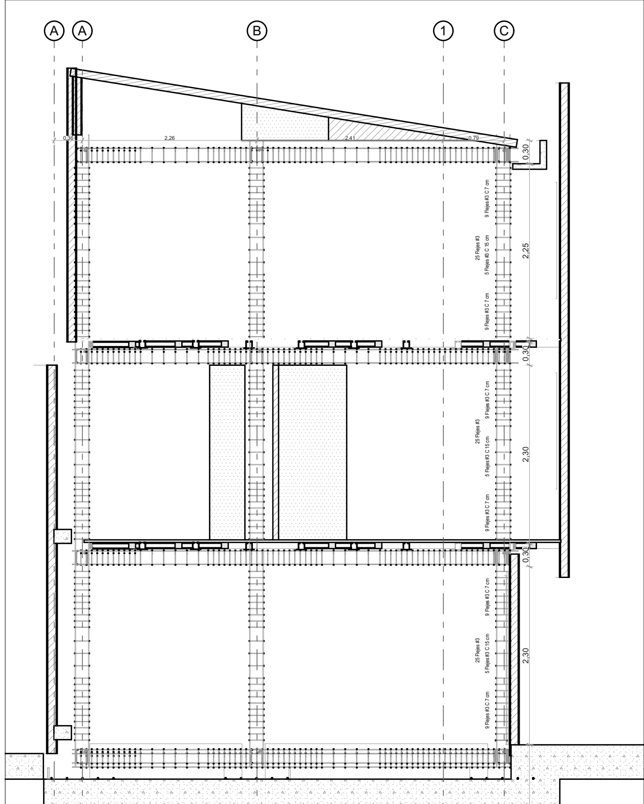
ALZADO LONGITUDINAL Esc 1: 50
