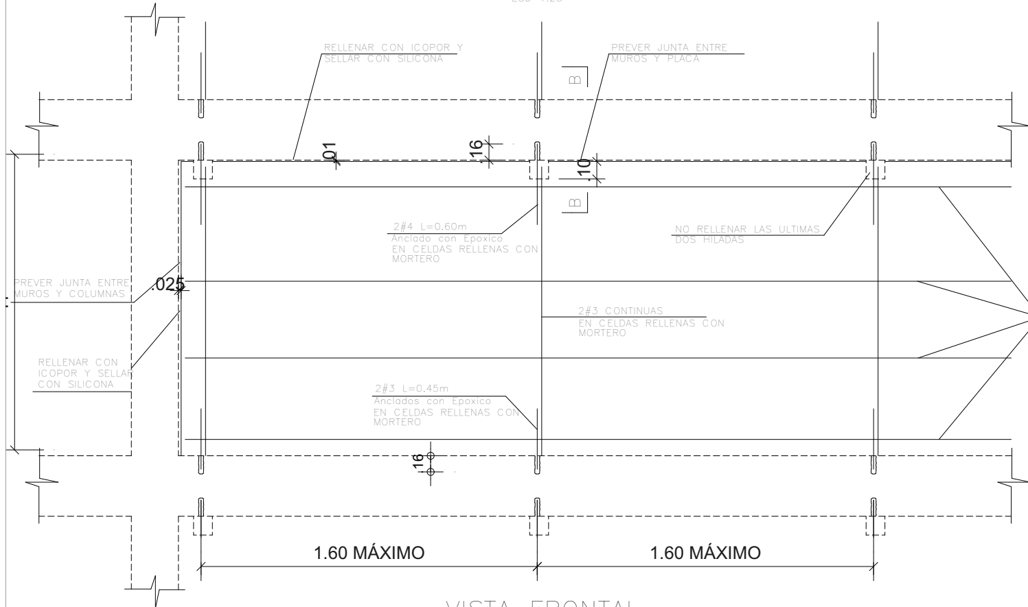
VISTA FRONTAL REFUERZO TÍPICO DE MUROS DE FACHADA DE ALTURA TOTAL EN LADRILLO TOLETE e = 0.25 \text{ m} ESC 1:25
