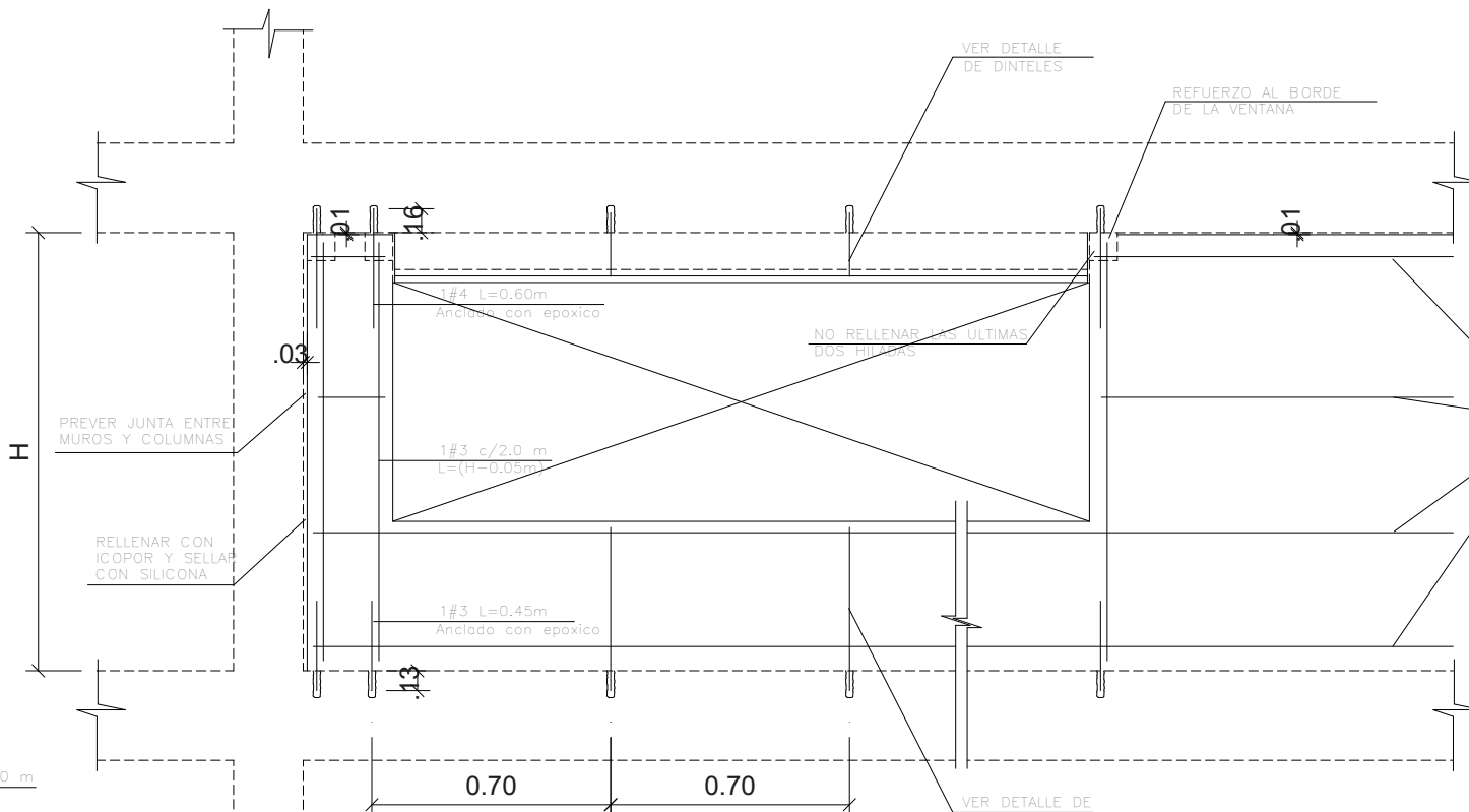
VISTA FRONTAL REFUERZO TÍPICO DE MUROS EN LADRILLO TOLETE e=0.15 \text{ m} CON ABERTURA ESC 1:25
