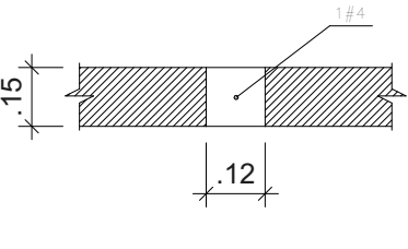
PARA MURO SENCILLO ESC 1:12.5
