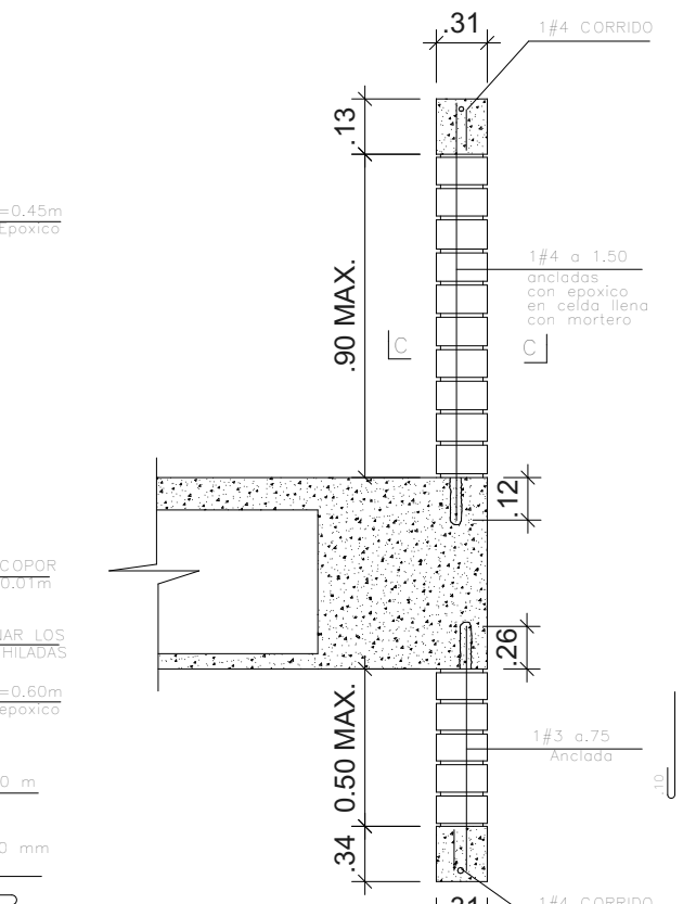
DETALLE DE DINTELES Y ANTEPECHOS EN LADRILLO TOLETE ESC 1:12.5
