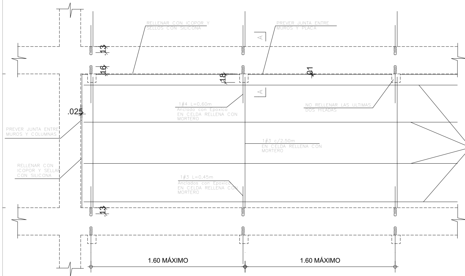
VISTA FRONTAL REFUERZO TÍPICO DE MUROS DE FACHADA DE ALTURA TOTAL EN LADRILLO TOLETE e = 0.15 \text{ m} ESC 1:25
