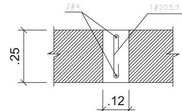
PARA MURO DOBLE ESC 1:12.5
