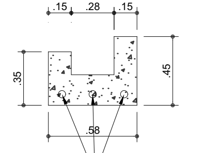
SECCIÓN VIGA CANAL 3#4
